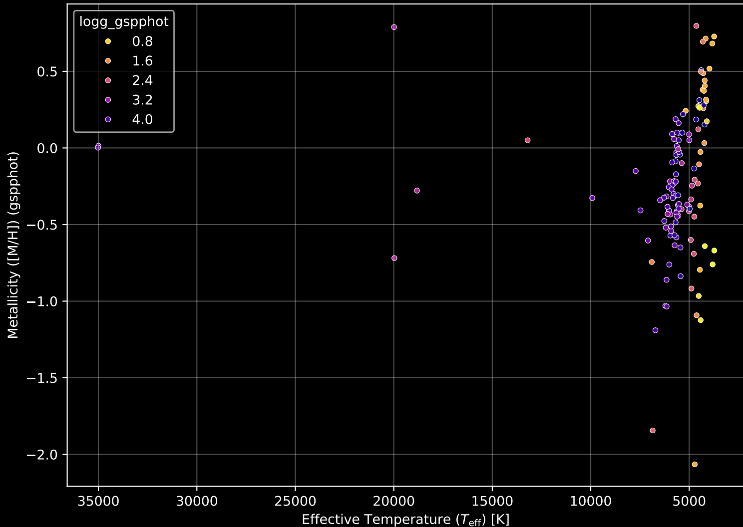
APOGEE DR17 Field: [279-31-O] Stellar Population Parameters (n= 125)
